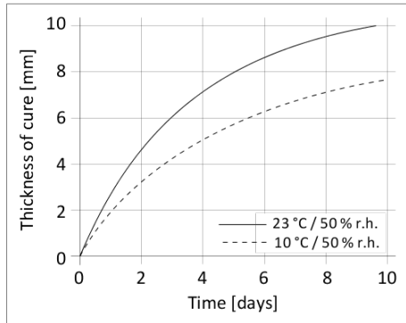
Diagramma 1: Velocità di indurimento per Sikaflex®-515
